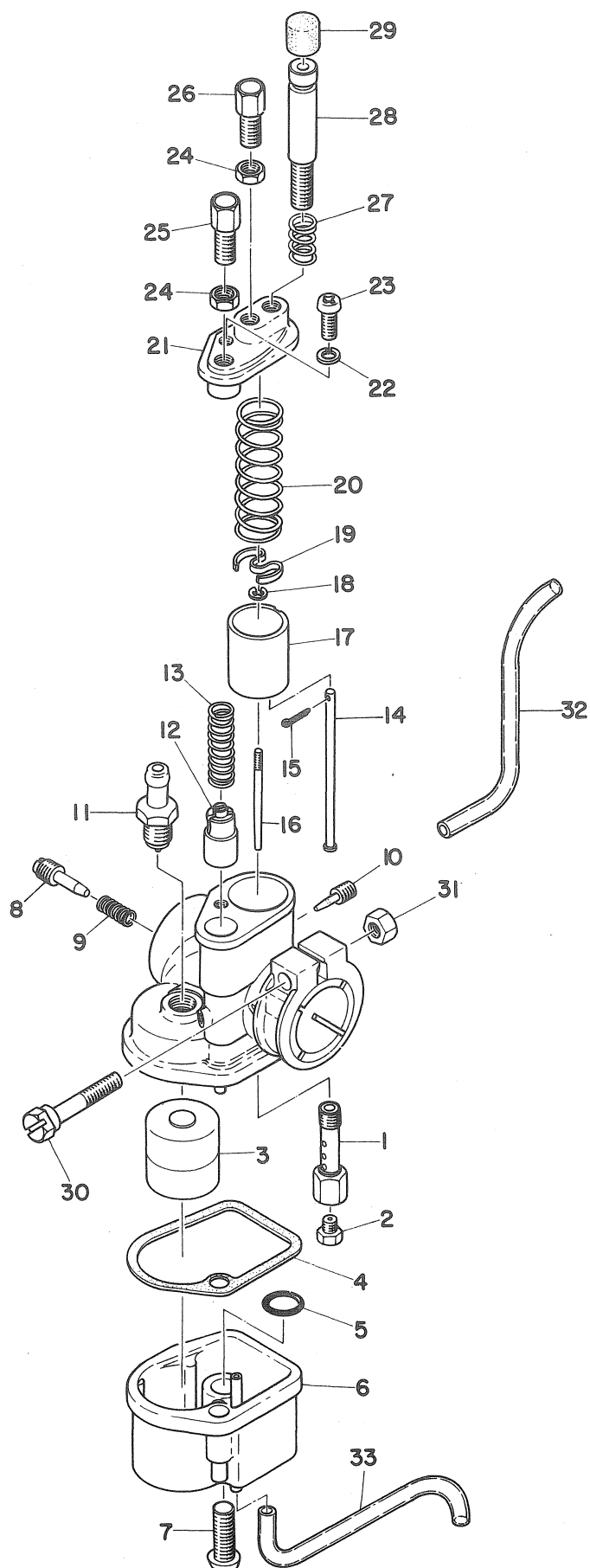
Fig. 10 CARBURETOR
