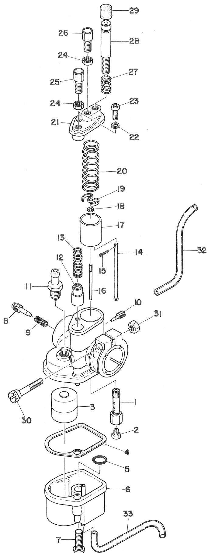
Fig. 10 CARBURETOR
