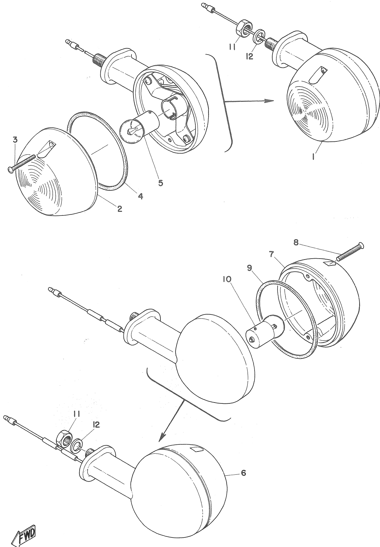
Fig. 28 FLASHER LAMP
