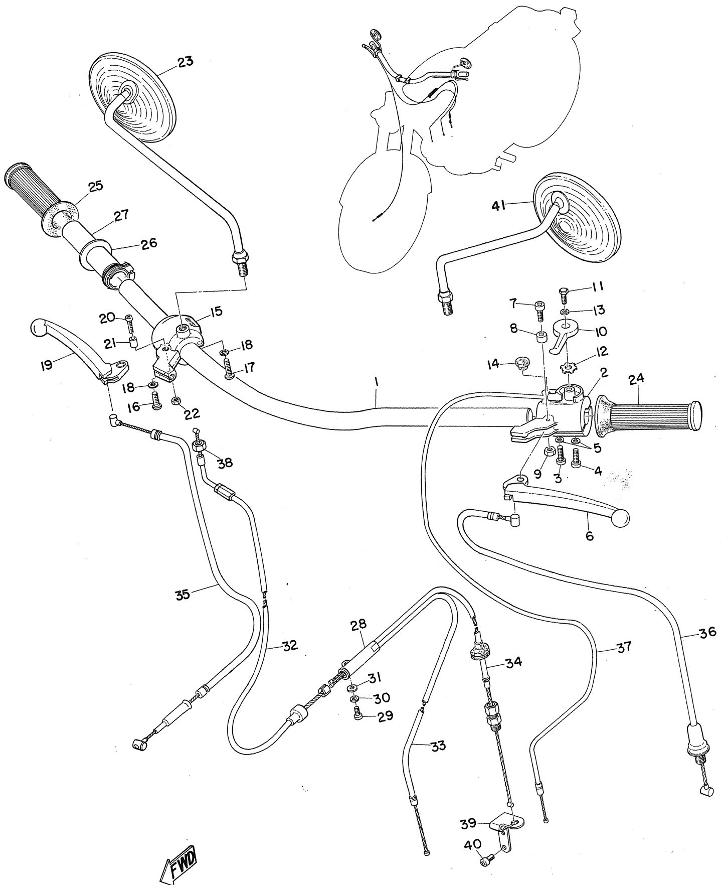
Fig. 19 HANDLE & WIRE
