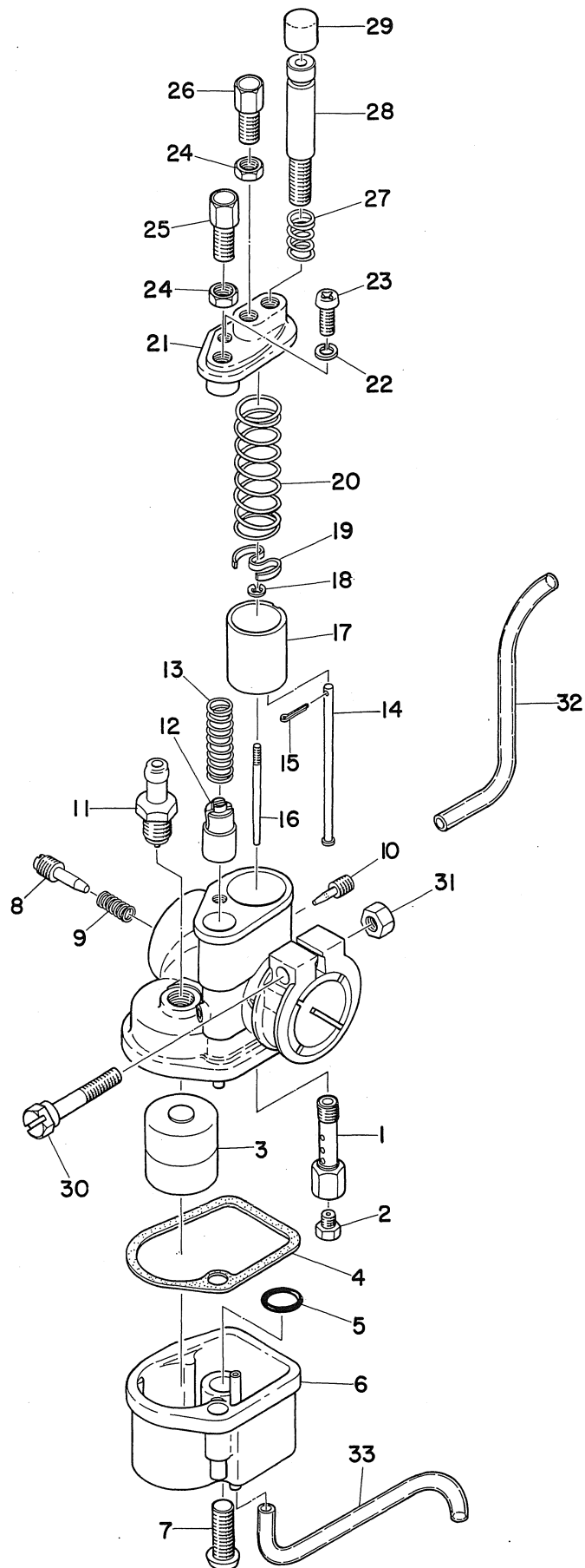
Fig. 10 CARBURETOR
