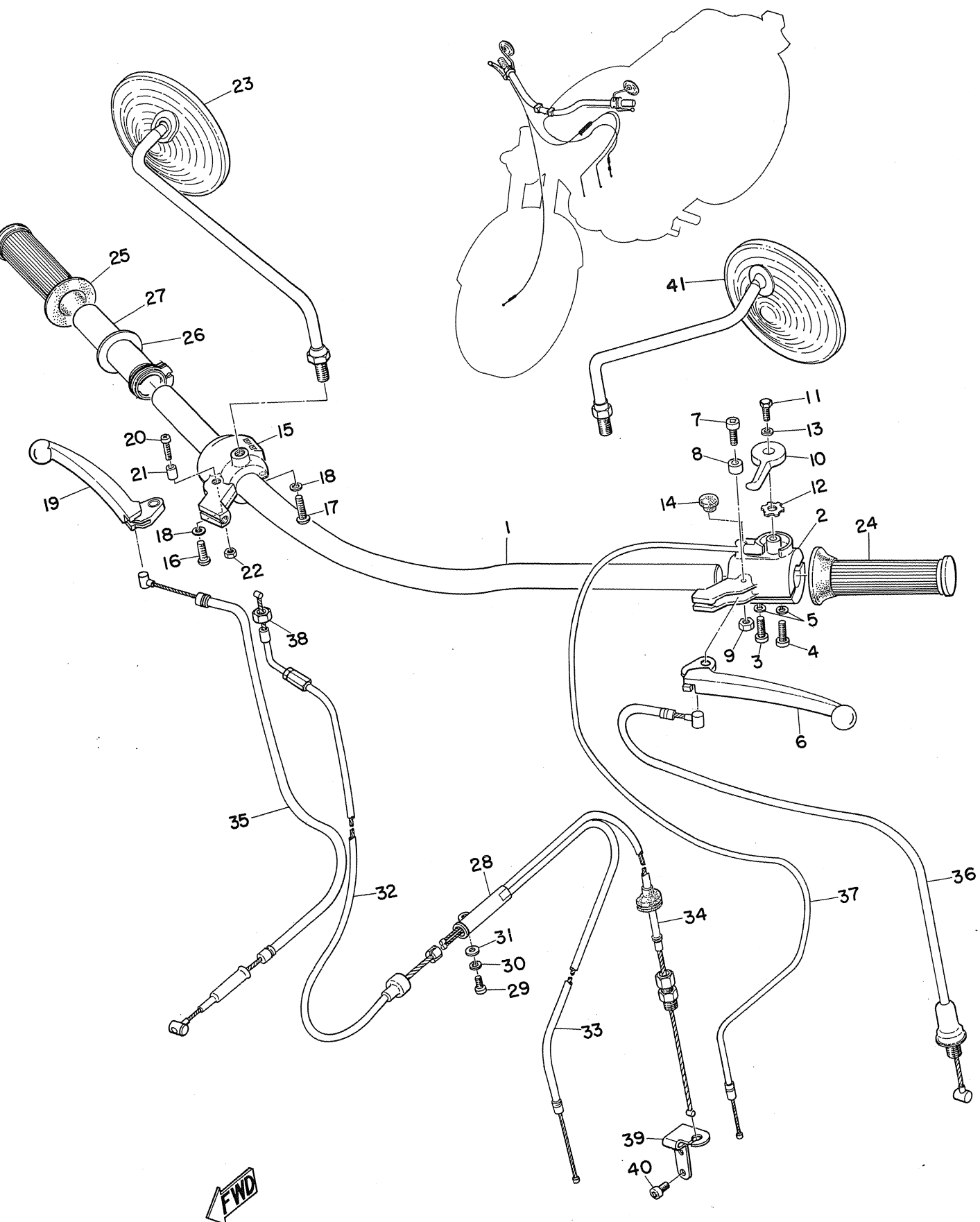
Fig. 19 HANDLE & WIRE
