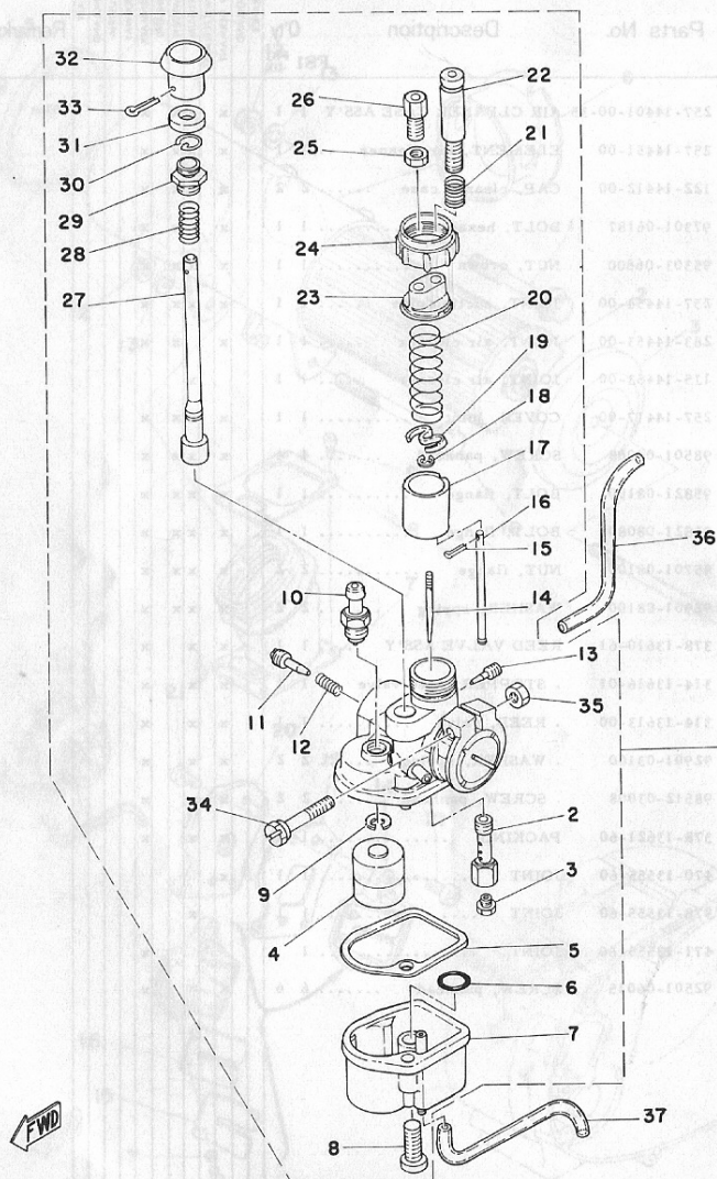
Fig. 10 CARBURETOR
