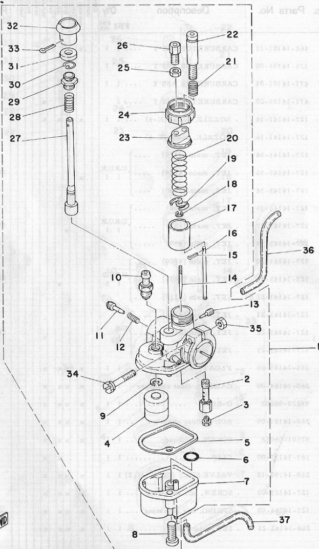
Fig. 10 CARBURETOR
