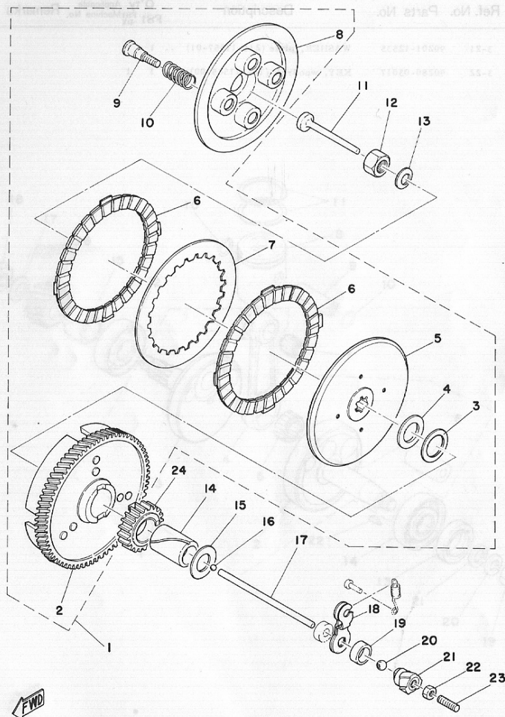
Fig. 4 CLUTCH
