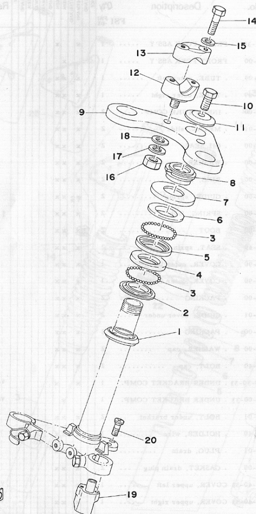
Fig. 19 STEERING
