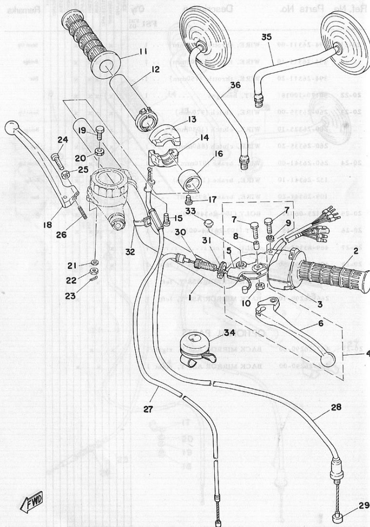
Fig. 21 HANDLE · WIRE
