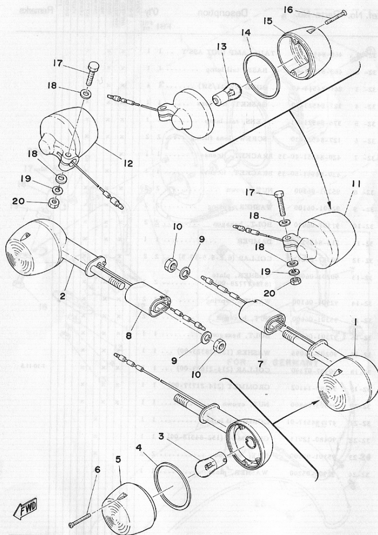
Fig. 33 FLASHER LAMP 1
