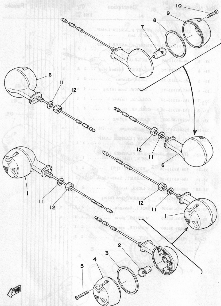
Fig. 34 FLASHER LAMP 2
