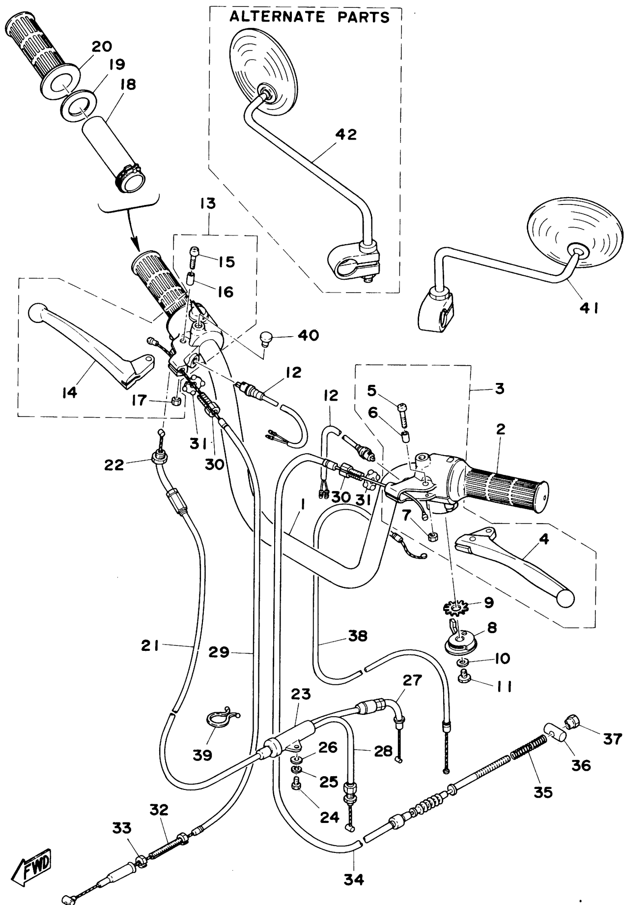
Fig. 19 HANDLE · WIRE
