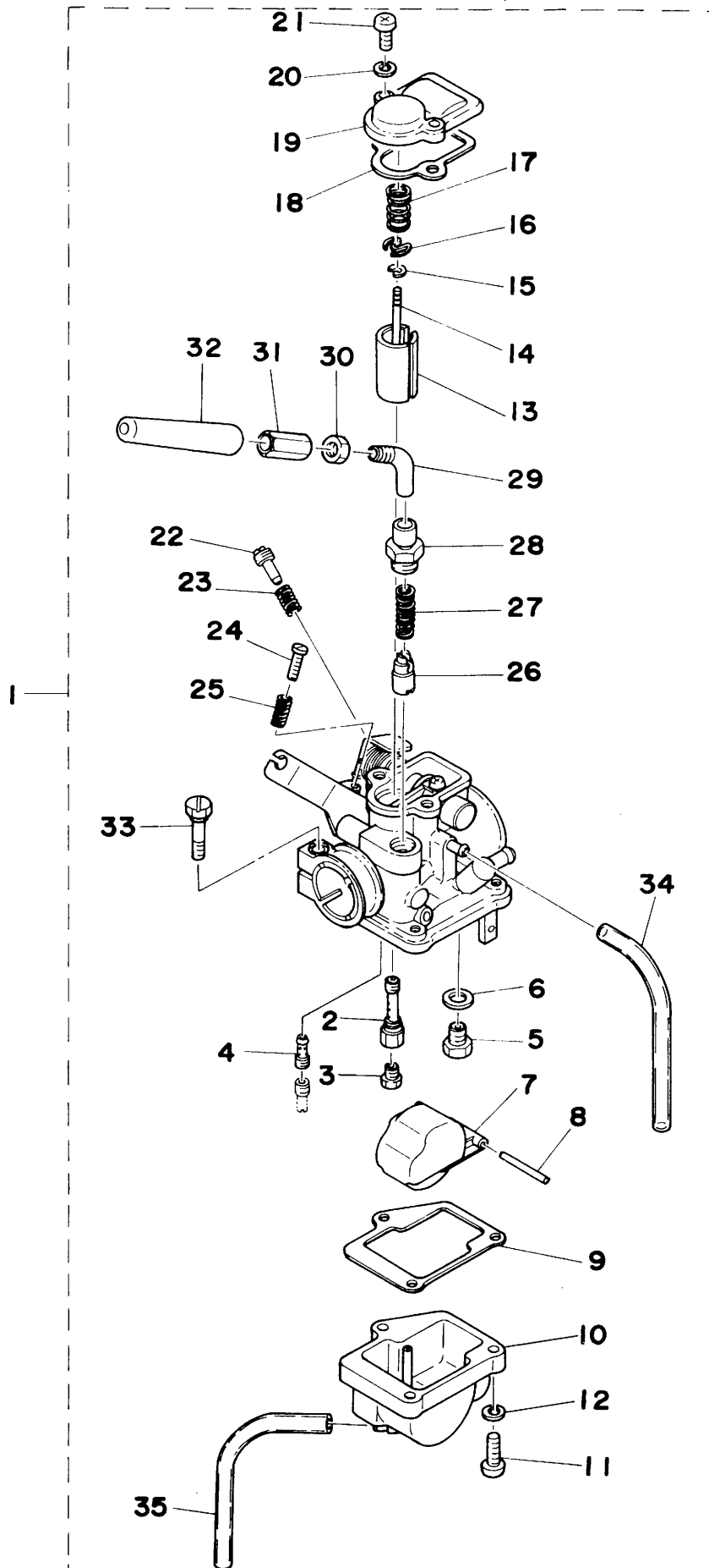
Fig. 9 CARBURETOR
