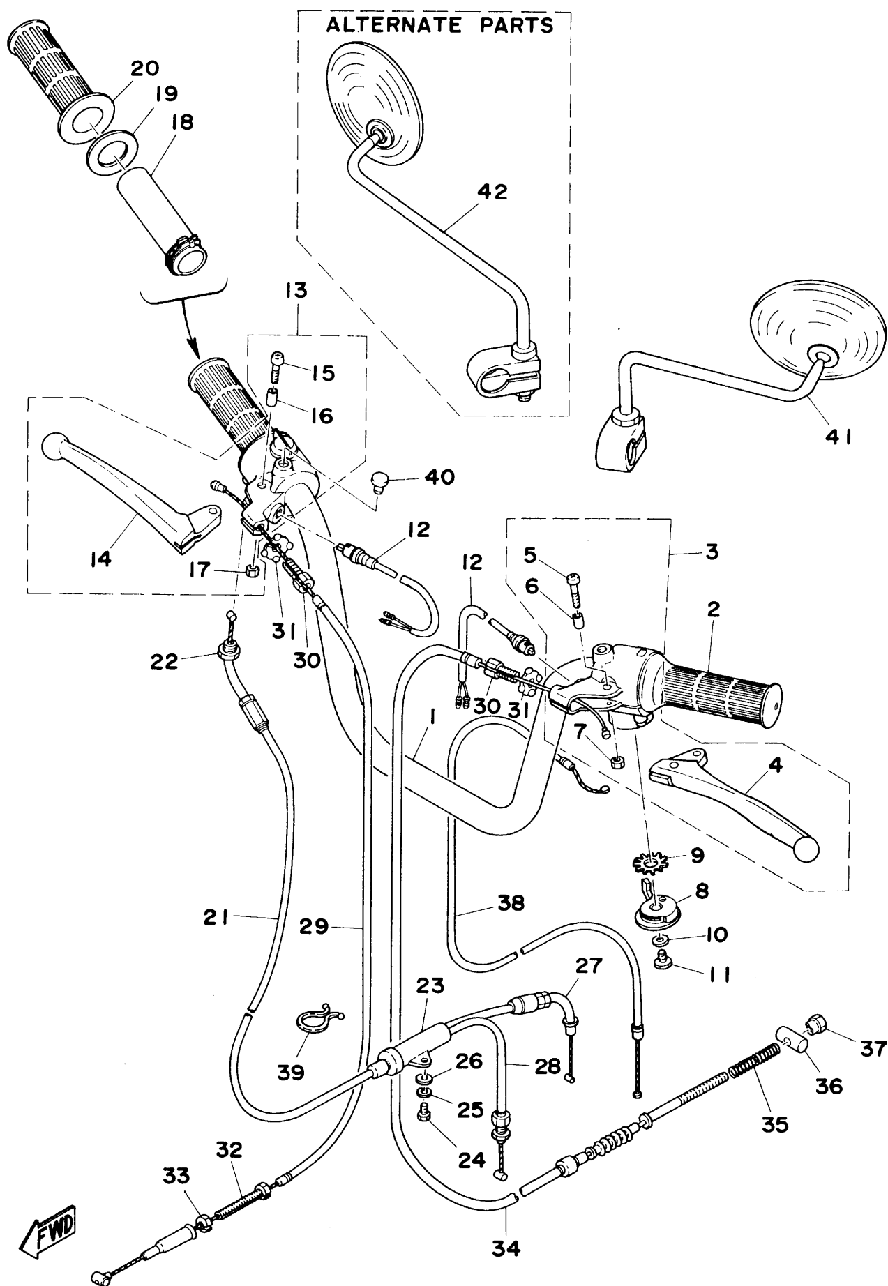
Fig. 19 HANDLE · WIRE
