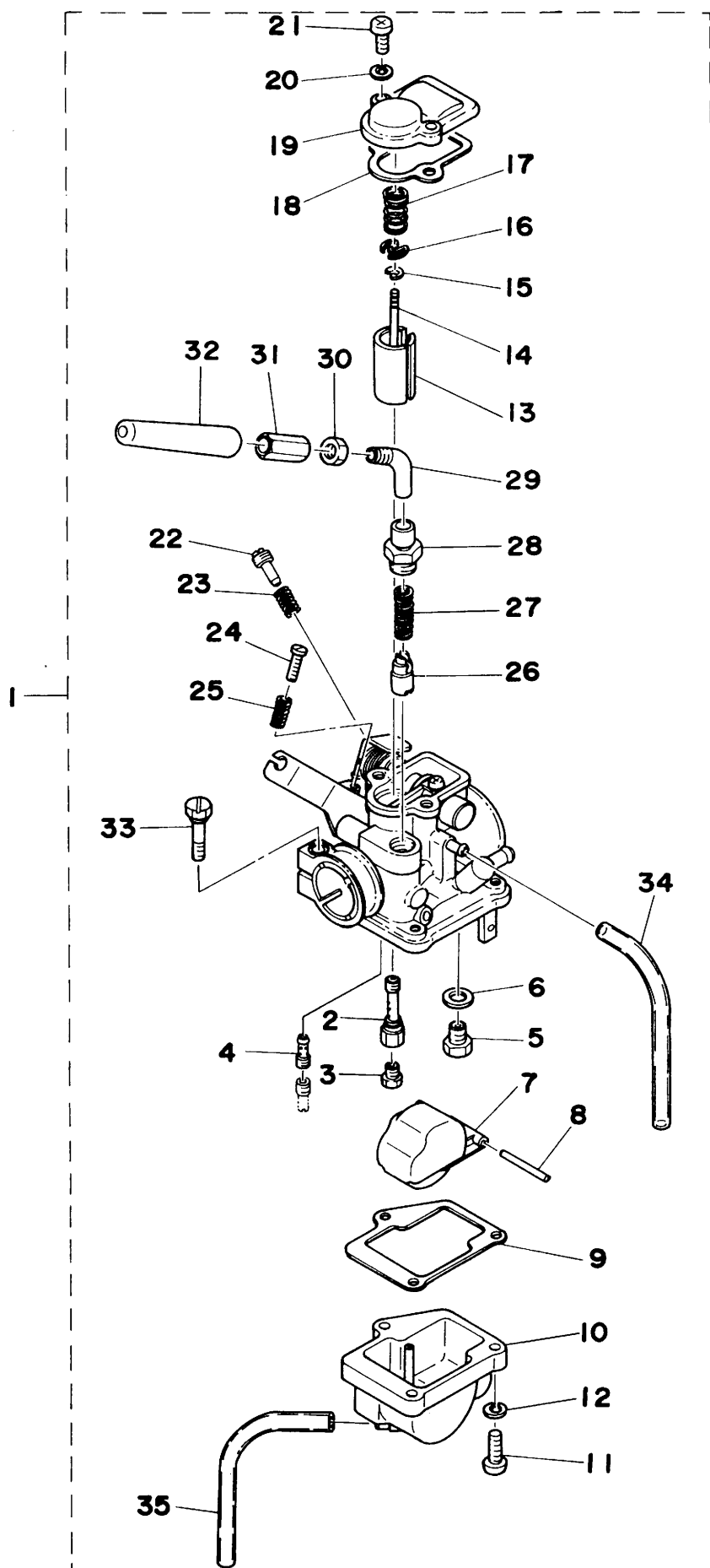
Fig. 9 CARBURETOR
