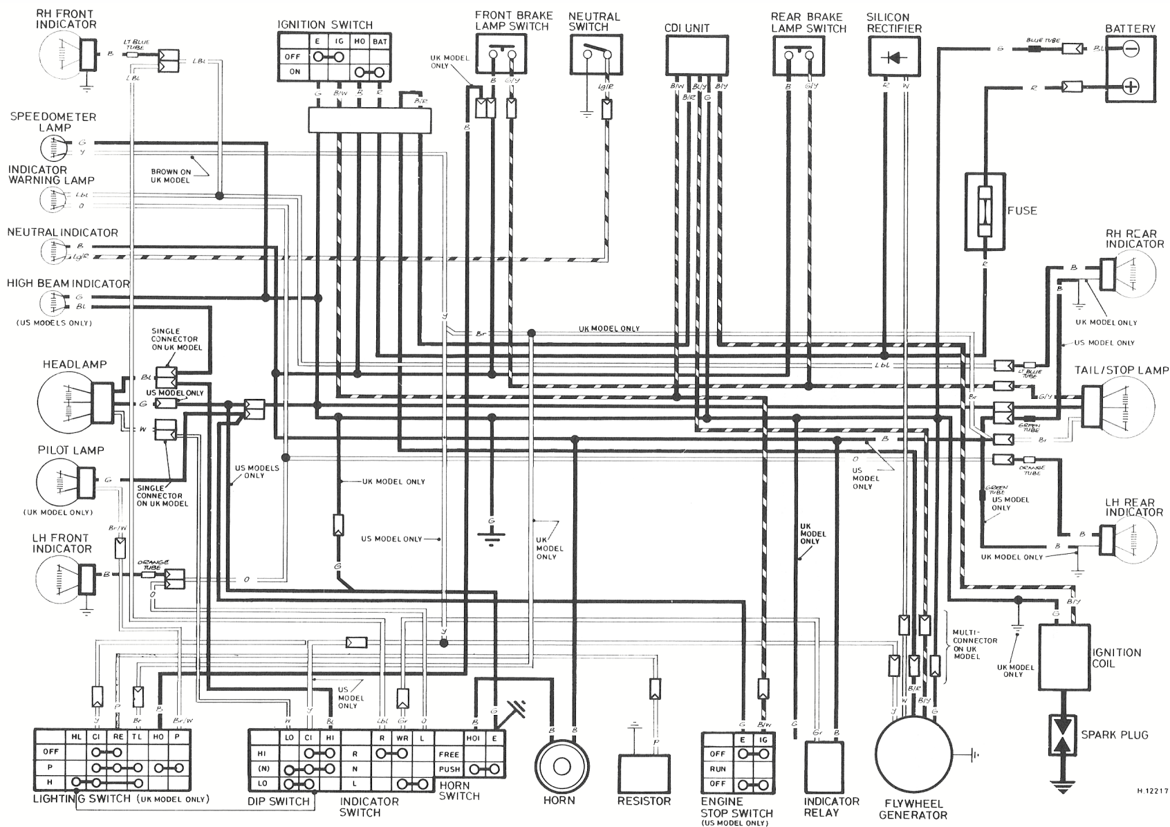
Wiring diagram – MB50 S-A and MB5
