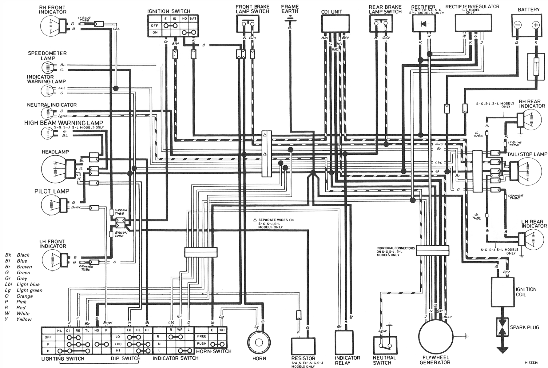
Wiring diagram - MT50 S-A, S-E/F, S-G, S-J and S-L
